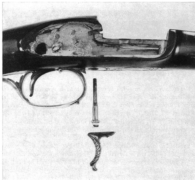
7. Nr 1820, det lösgjorda stödet framför varbygeln och den därunder sittande skruven med asymmetriskt huvud. — The support in front of the triggerguard and the screw with the asymmetric head.
